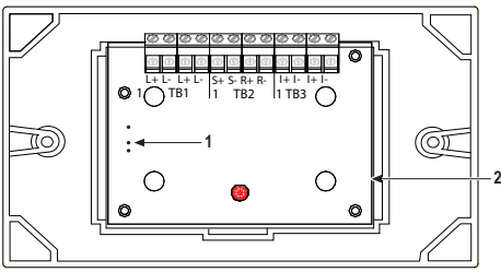
Fig. 2 FC410SNM colocado na cobertura. FC410SNM encaixada na cobertura.
