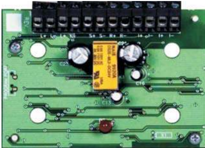
Fig. 1 Módulo de notificación de sirena FC410SNM
