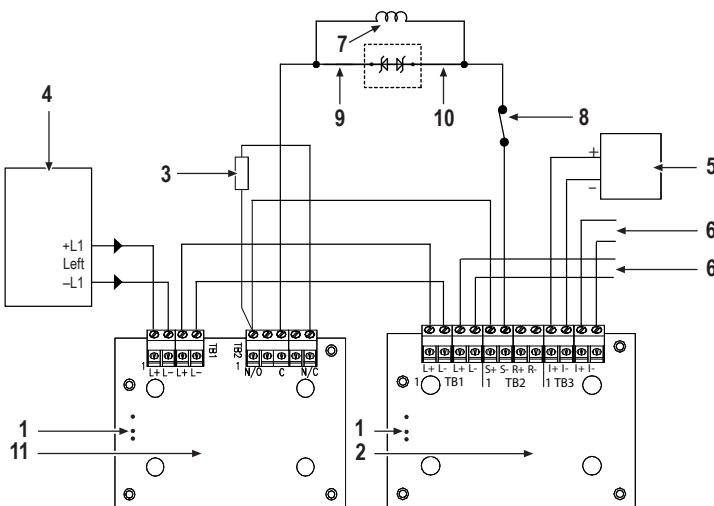
Fig. 6 Diagrama de conexões simplificado mostrando el FC410SNM conectado en una configuración para activación de dispositivos de extinción. Diagrama simplificado de cabeamento mostrando o FC410SNM conectado em uma configuração de liberação de extincção.
