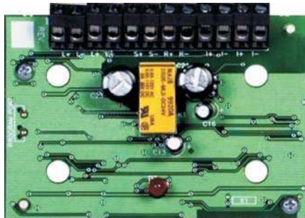
Fig. 1 Módulo de notificação de alarme sonoro FC410SNM
