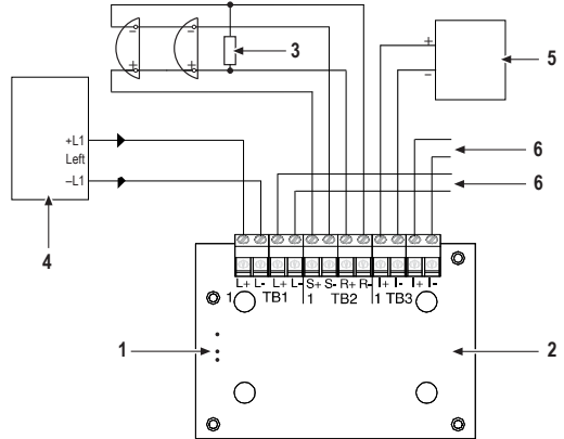
Fig. 5 Diagrama de conexões simplificado mostrando sirenas conectadas em configuração de laço. Diagrama simplificado de cabeamento mostrando os alarmes sonoros conectados a uma configuração de circuito.
